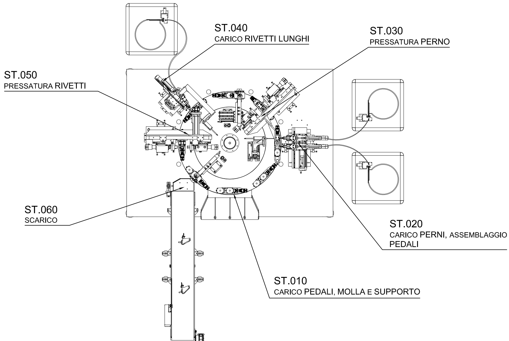
IMPIANTO SEMIAUTOMATICO DI ASSEMBLAGGIO FRENI SU SUPPORTI
